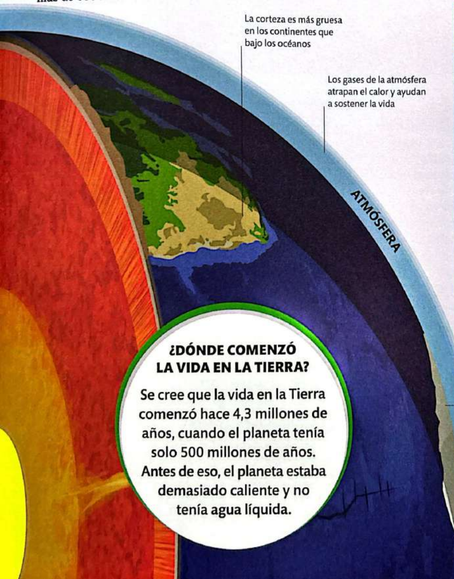
OCEANO EN FORMACIÓN
