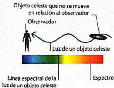
OBSERVADOR Y OBJETO ESTACIONARIOS
