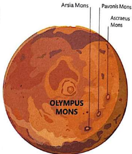
ABULTAMIENTO DE THARSIS DESDE ARRIBA
