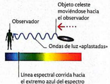
OBSERVADOR Y OBJETO ACERCÁNDOSE ENTRE SÍ
