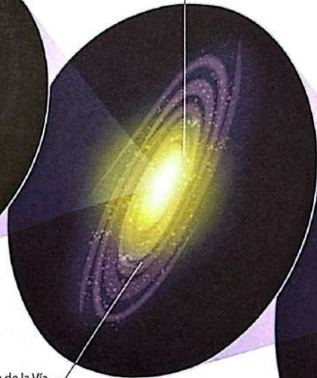
LA VÍA LÁCTEA
